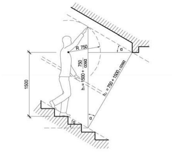
Obrázek 4: Nejmenší dovolená podchodná ( h_1 ) a průchodná ( h_2 ) výška
